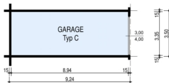
GRUNDRISS
